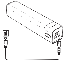
圖2：Type-c口給移動電源充電
